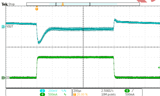
图 19 负载响应 (从 0 到 1A, 0.25 A/\mu s 变换率)
